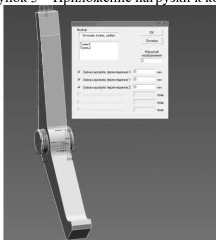
Рисунок 4 – Закрепление колена
